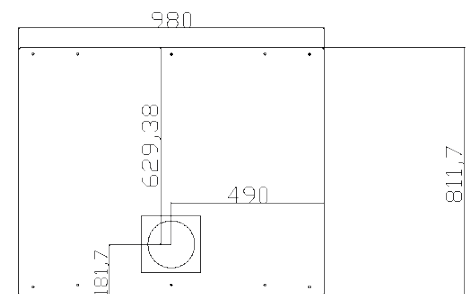
Κάτοψη/ Top view
