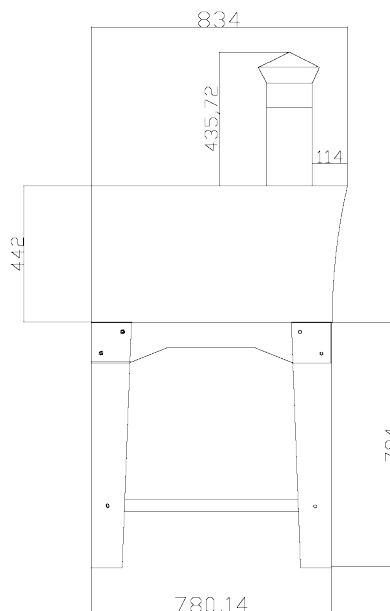
Πλάγια όψη/ Side view
